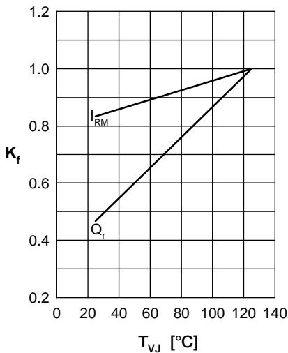
Fig. 4 Dyn. parameters K_f , I_{RM} , Q_r versus T_{VJ}
